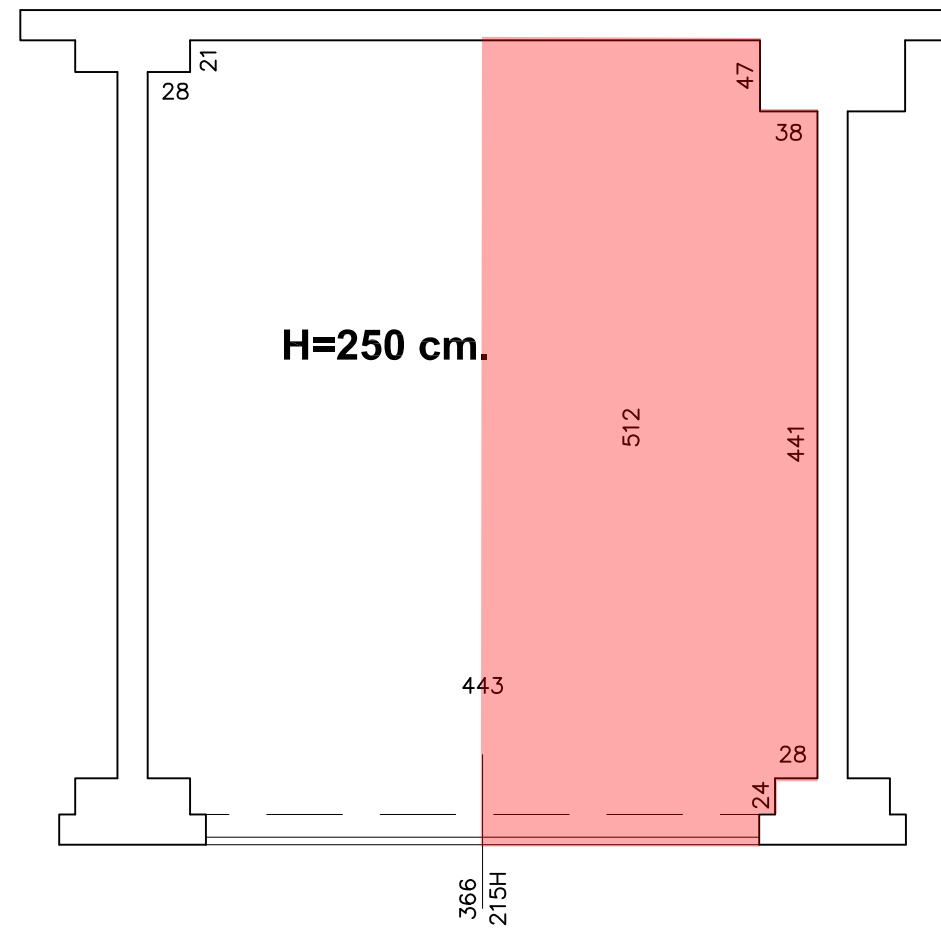
AUTORIMESSA VIA PRUDENZIANA 10 - COMO PIANO - 1
