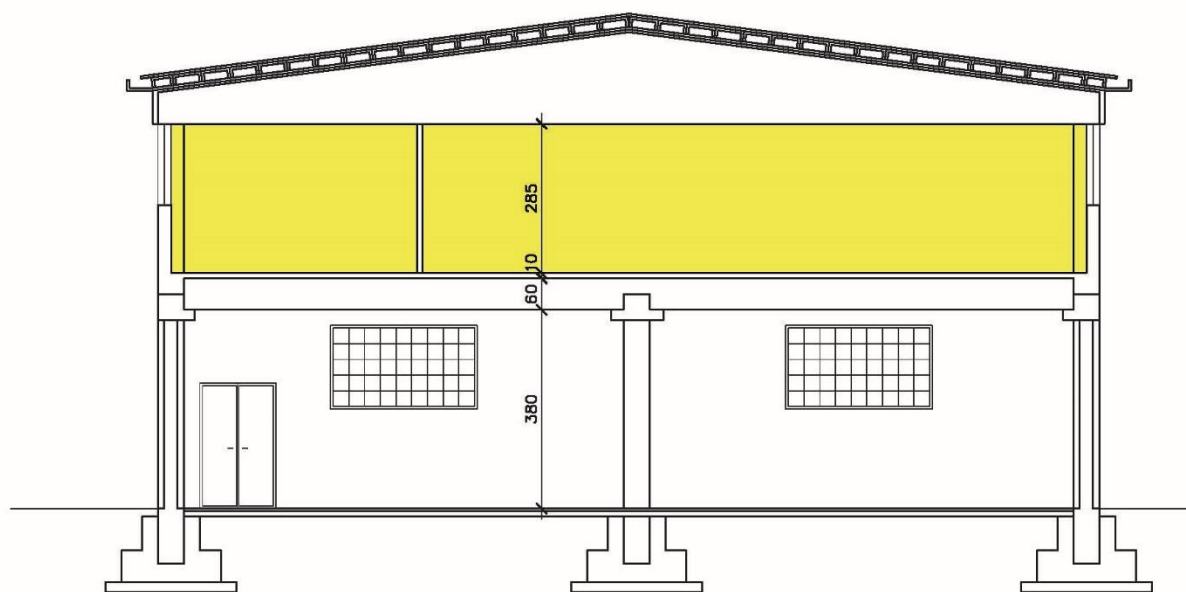
SEZIONE A-A 1 : 100
